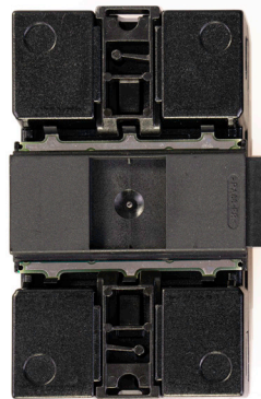
Abb.: Solar-Log Base / Solar-Log MOD I/O mit Busverbinder
